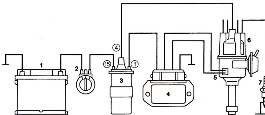
Elementy składowe układu elektronicznego
