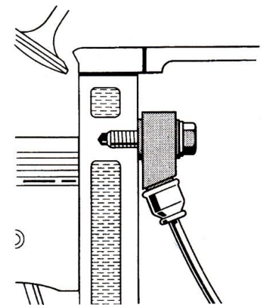
Czujnik spalania stukowego
