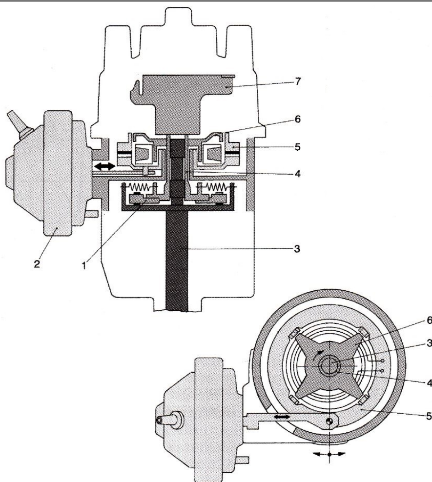
Schemat współdziałania regulatora podciśnieniowego i odśrodkowego przy sterowaniu zapłonu przez czujnik indukcyjny
