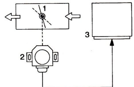
Czujnik spalania stukowego
