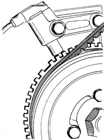
Koło zębate z czujnikiem indukcyjnym
