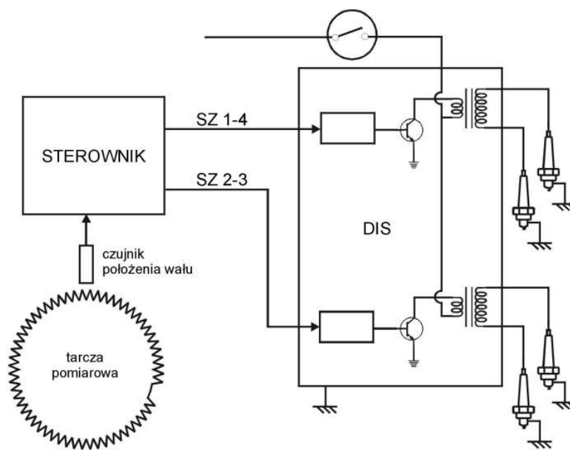
Schemat połączeń modułu zapłonu DIS ze sterownikiem
