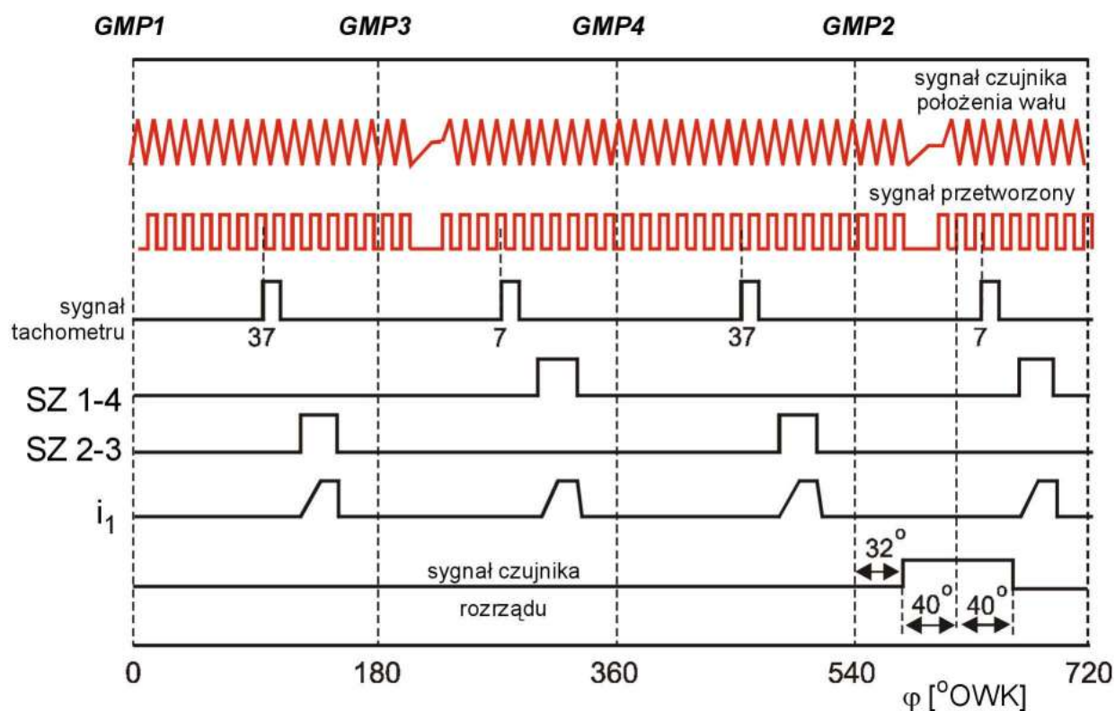
Przebieg sygnałów podczas pracy układu zapłonowego sterowanego z poziomu sterownika centralnego sygnałami SZ 1-4 i SZ 2-3
