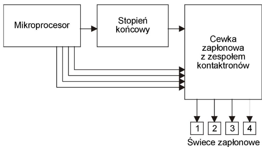
Schemat bezrozdzielaczowego układu zapłonowego z kontaktronami
