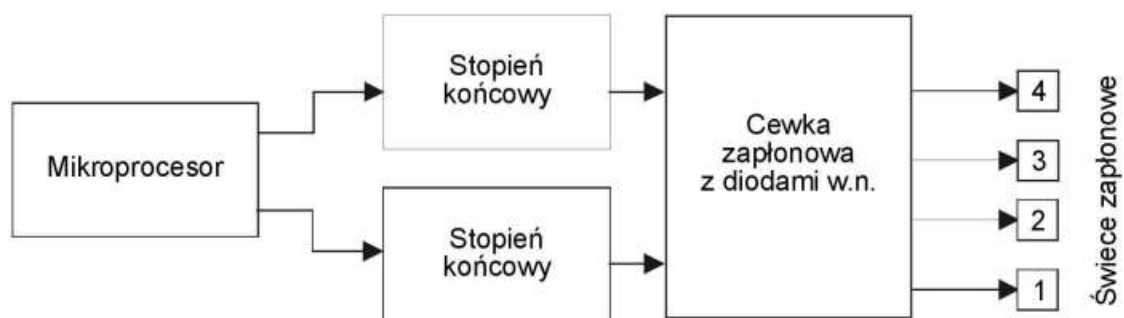
Schemat bezrozdzielaczowego układu zapłonowego z jedną cewką i diodami
