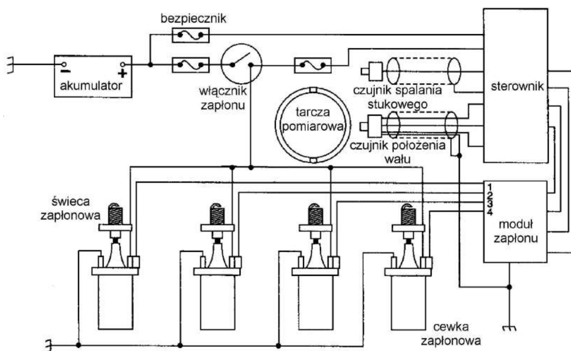
Schemat połączeń bezrozdzielaczowego modułu zapłonowego
