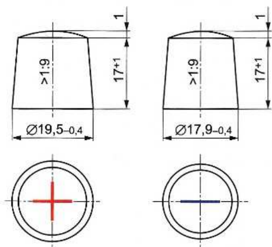
Rys. 4.2. Kształt i podstawowe wymiary zacisków akumulatora
