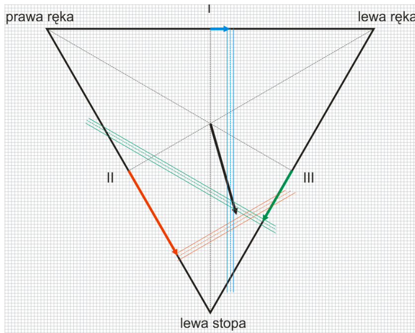
Ryc. 4. Schemat wykreślania osi elektrycznej serca a) fotografia elektrokardiogramu z zaznaczonymi załamkami QRS, które były wzięte do wykreślenia osi elektrycznej serca, b) wykreślona na papierze milimetrowym oś elektryczna serca w skali 4:1, z zaznaczeniem niepewności odczytu rzutów chwilowego wektora elektrycznego, uśrednionego w czasie depolaryzacji komórek, na osie odpowiednich odprowadzeń.
